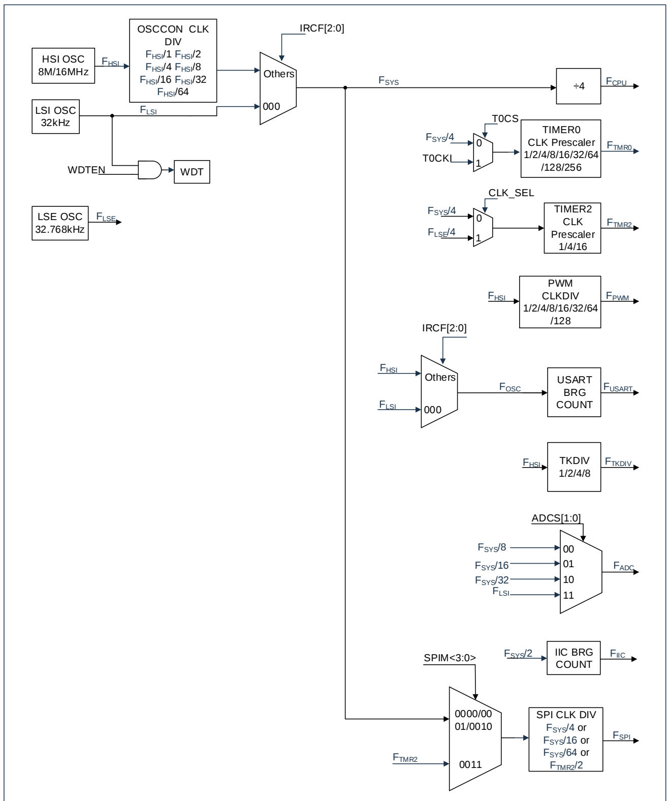
图 3-2: 时钟框图
